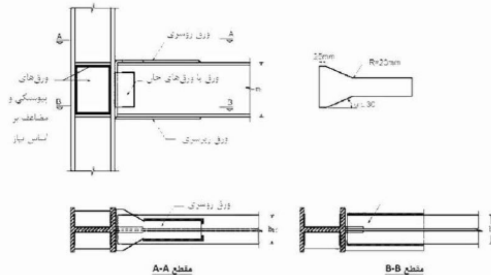
شکل ۱-۳-۷-۶: اتصال گیردار جوشی به کمک ورق های روسری و زیرسری (WFP)
