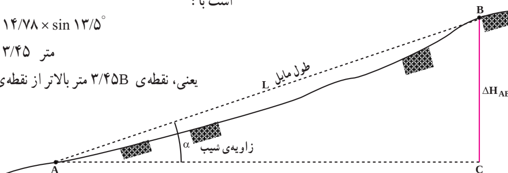
شکل ۸-۳- ترازیابی غیرمستقیم
