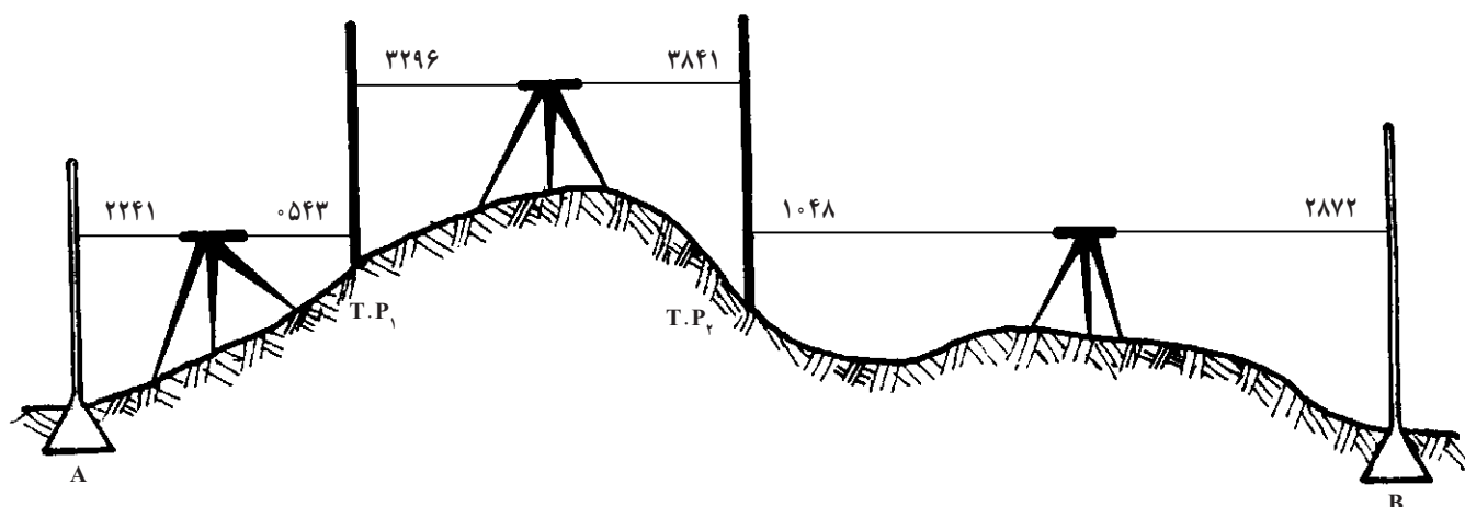
شکل ۳۹-۸- ترازبابی تدریجی
