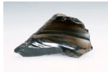
شیل (Shale)
